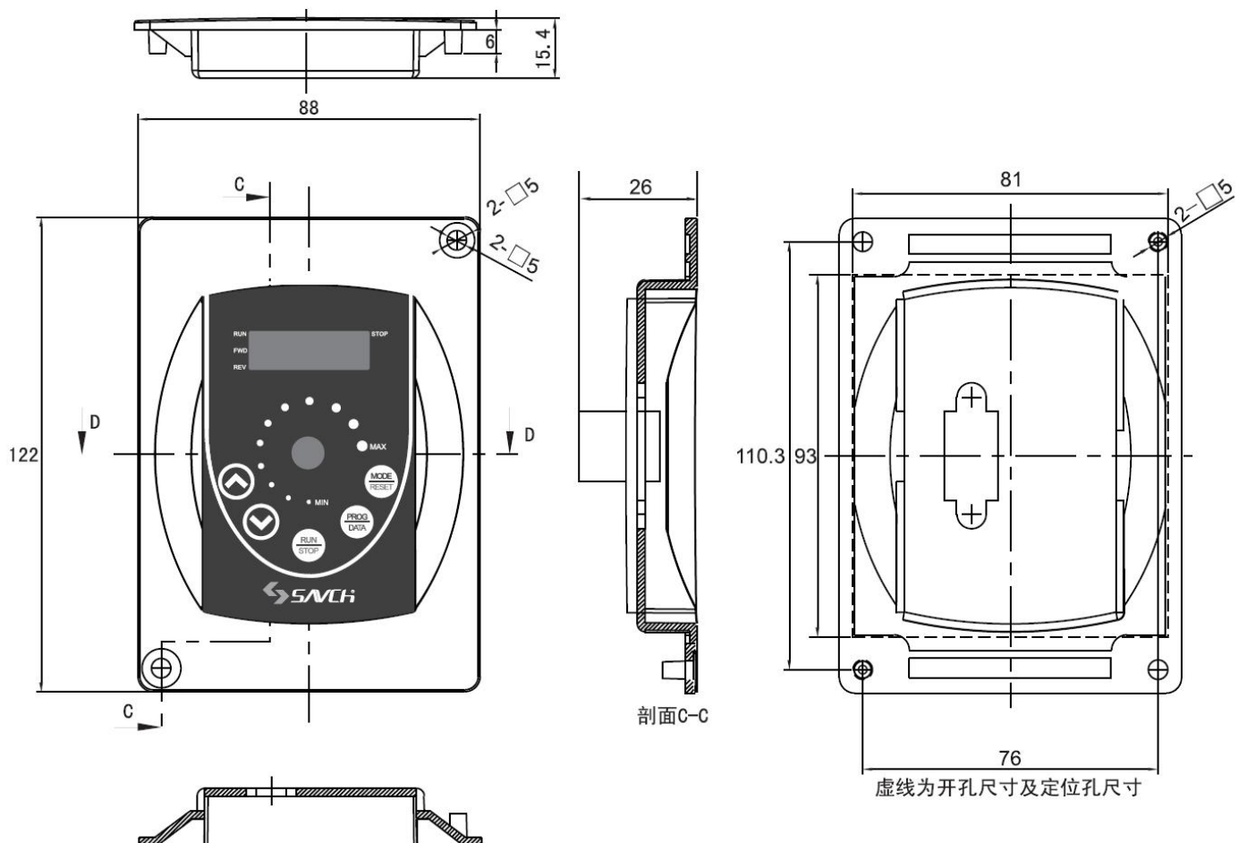
操作器外形尺寸及安装孔尺寸
