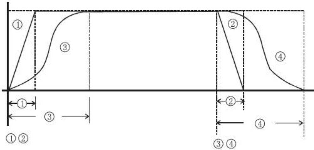
无 S 曲线时之加/减特性
