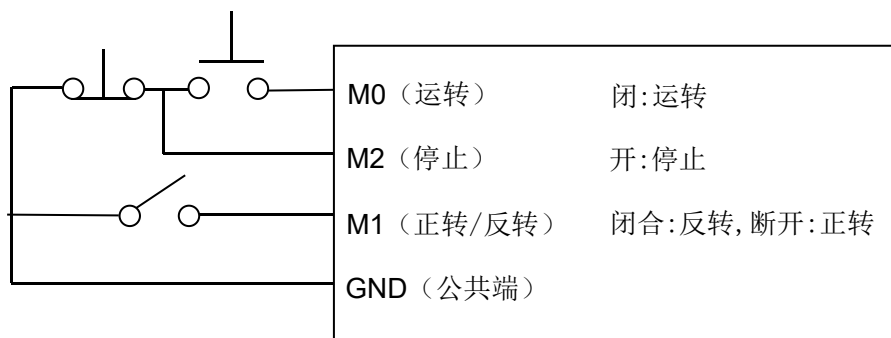
三线式控制（1）
