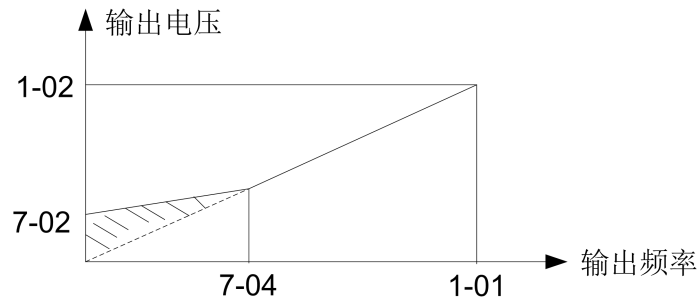
手动转矩提升（提升量为阴影部分）
