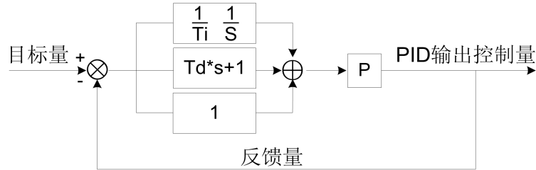
图 5-25 过程 PID 原理框图
