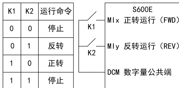
图 5-6 两线式模式 1
