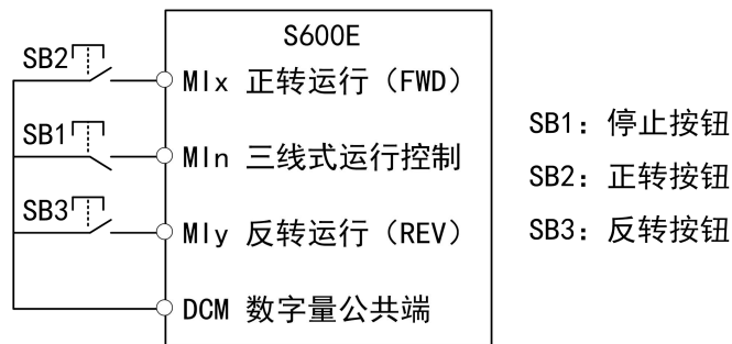
图 5-8 三线式控制模式 1
