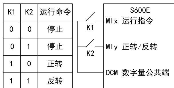
图 5-7 两线式模式 2
