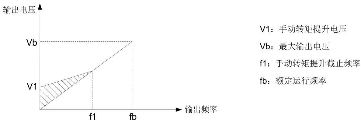
图 5-3 手动转矩提升示意图
