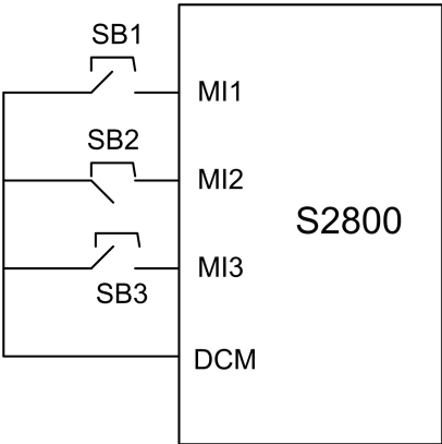
三线式控制模式 2
