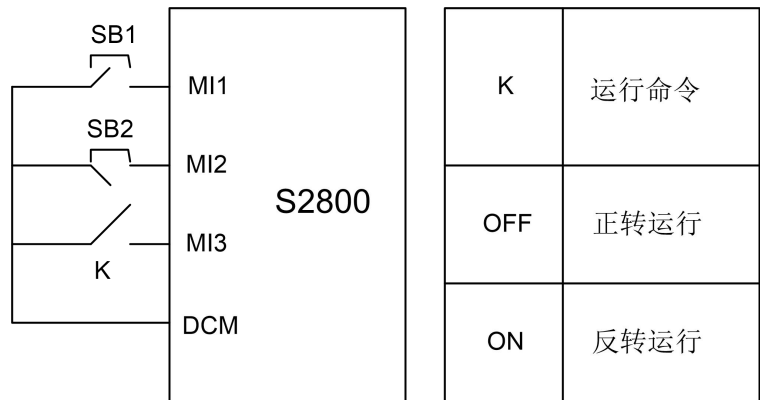
三线式控制模式1
