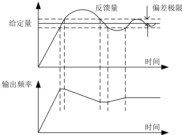
偏差极限与输出频率的对应关系
