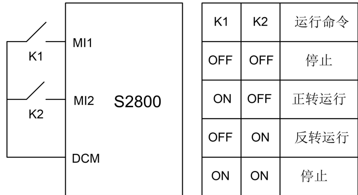
两线式控制（使能与方向合一）
