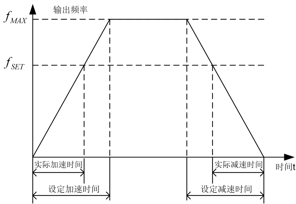
加减速时间示意图
