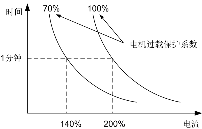
电机过载保护系数设定
