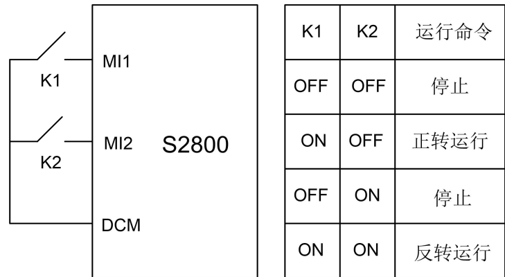
两线式控制（使能与方向分离）
