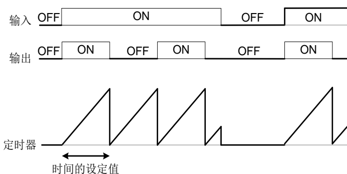
(5) 脉冲串输出
