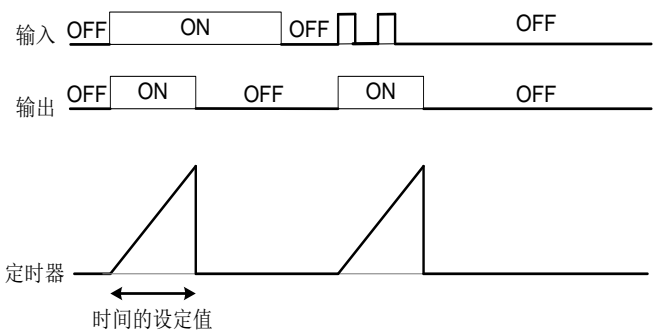
(3) 脉冲
