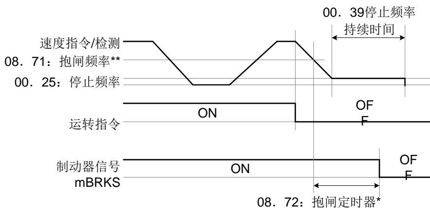
·抱闸条件选择（位4）：1（运转指令OFF有效）的时序图
