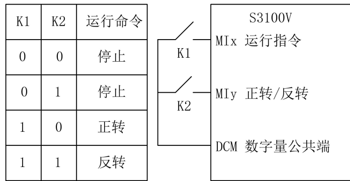
图 5-7 两线式模式 2
