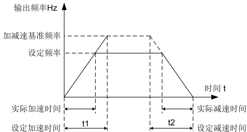
图 5-1 加减速时间示意图
