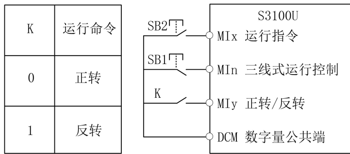
SB1: 停止按钮 SB2: 运行按钮
