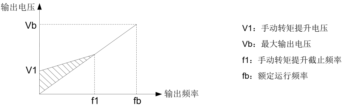
图 5-3 手动转矩提升示意图
