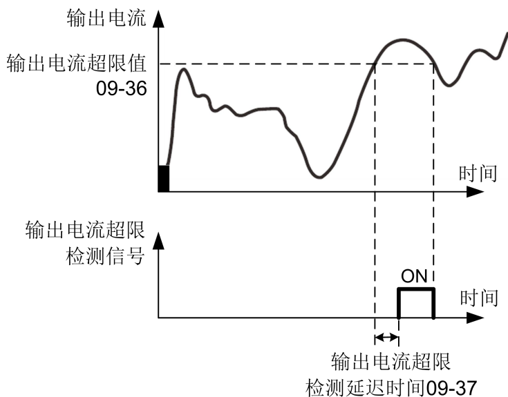
图 5-23 输出电流超限检测示意图
