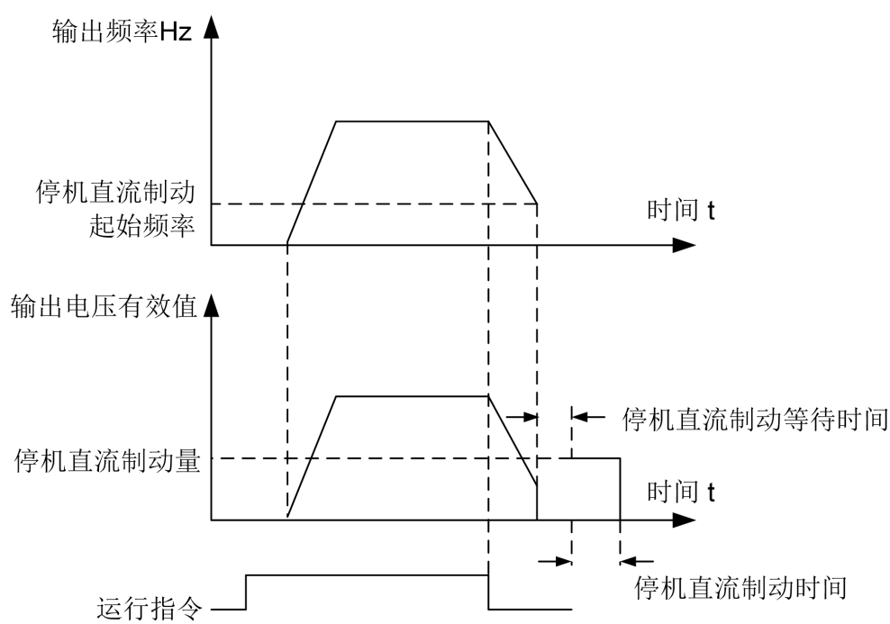
图 5-12 停机直流制动示意图
