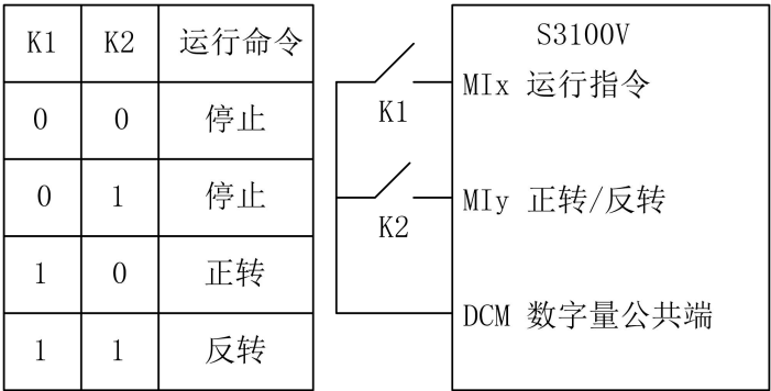
图 5-7 两线式模式 2
