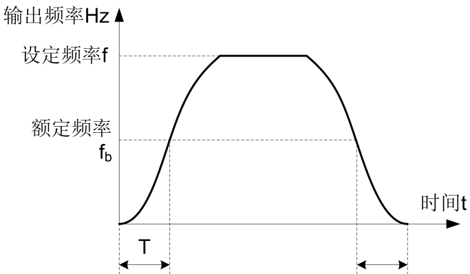
图 5-14 S 曲线加减速 B 示意
