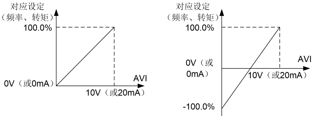
图 5-10 模拟给定与设定量的对应关系
