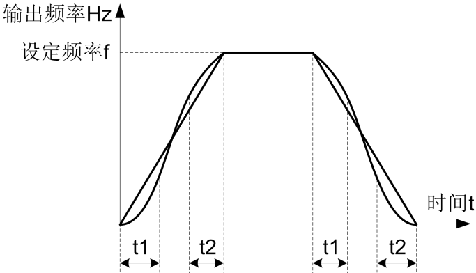
图 5-13 S 曲线加减速 A 示意
