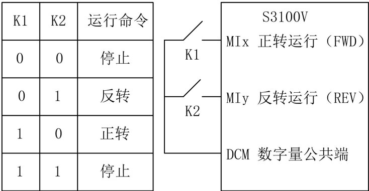
图 5-6 两线式模式 1
