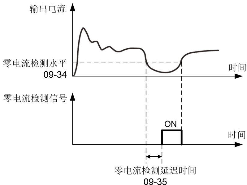
图 5-22 零电流检测示意图
