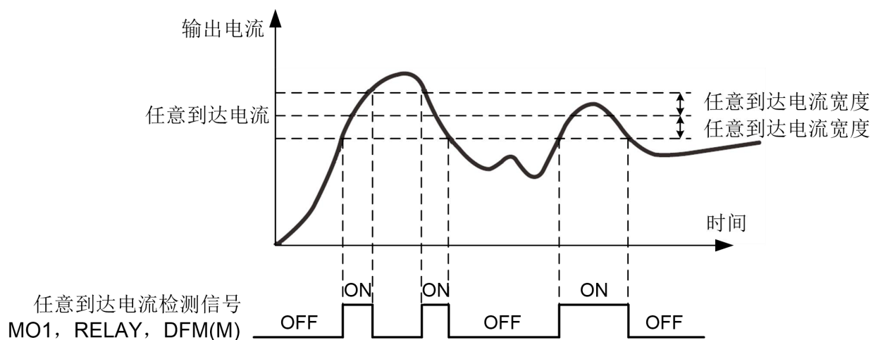
图 5-24 任意到达电流检测示意图
