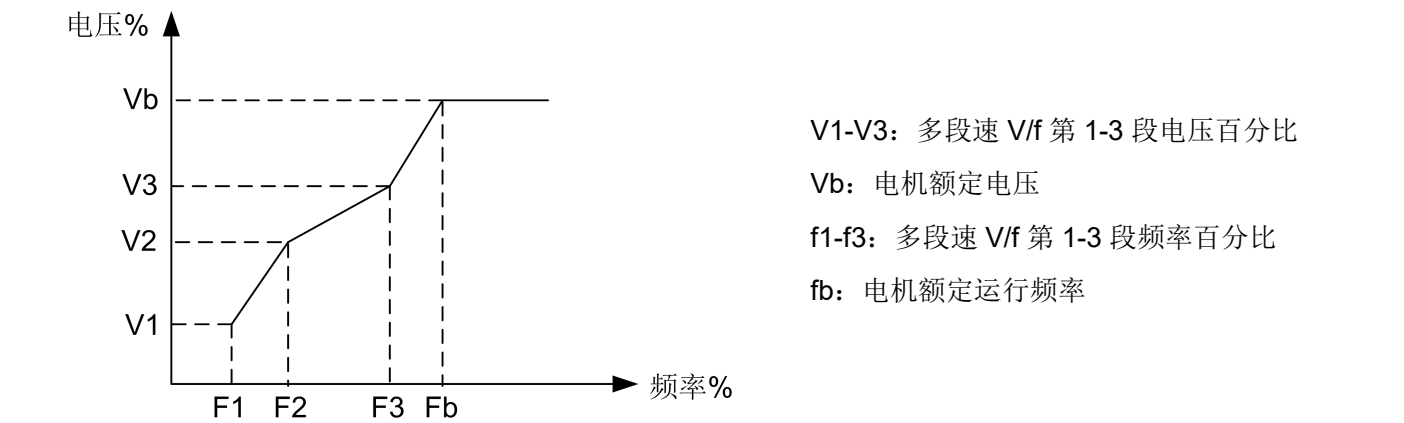
图 5-4 多点 V/f 曲线设定示意图
