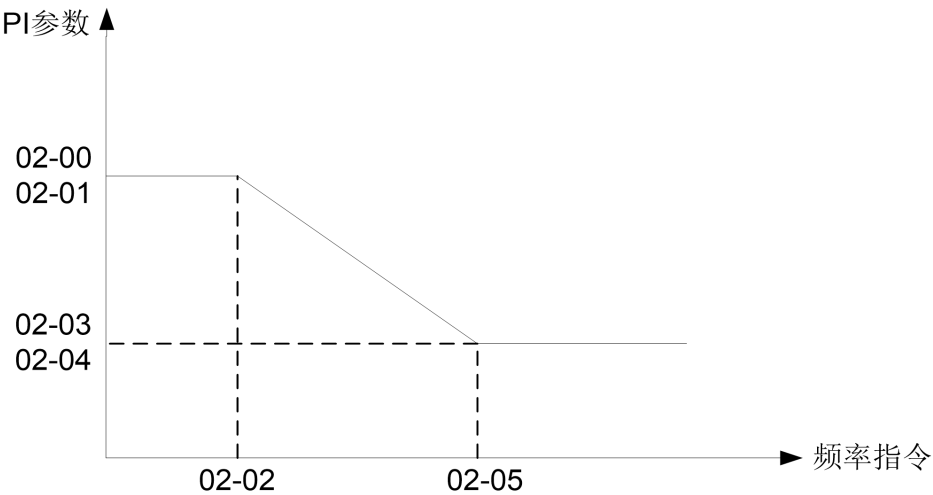
图 5-2 PI 参数示意图
