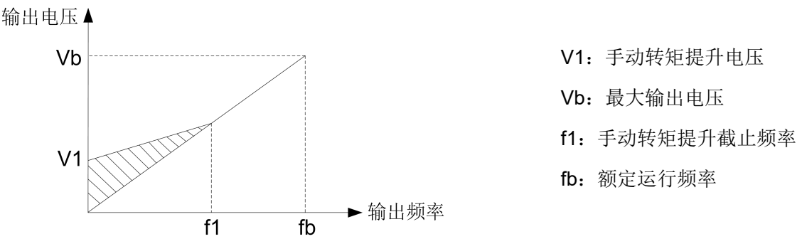
图 5-3 手动转矩提升示意图
