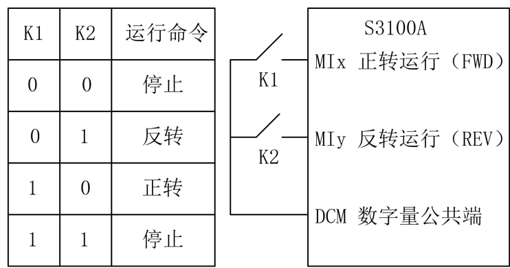
图 5-6 两线式模式 1
