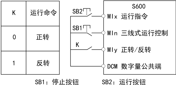
图 5-9 三线式控制模式 2
