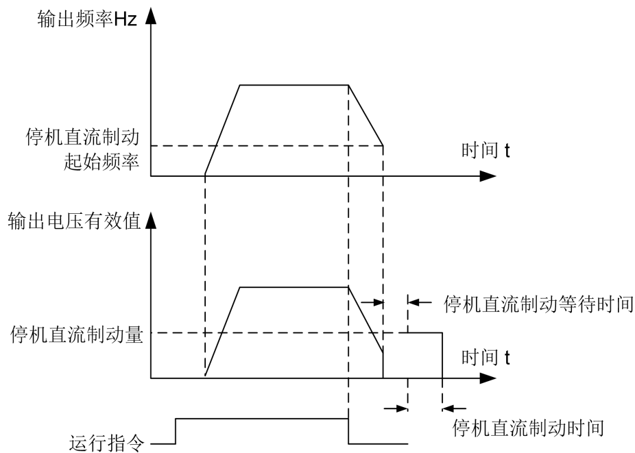
图 5-12 停机直流制动示意图
